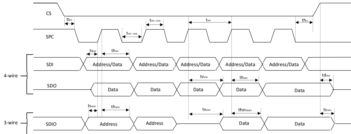
SPI : Mode 3
